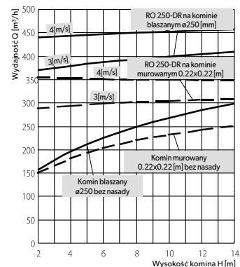
Wykres wydajności samonastawnych nasad kominowych ROTOWENT DRAGON ø250 dla kominia blaszanego i muranego, dla dwóch prędkości wiatru 3 i 4 [m/s].
