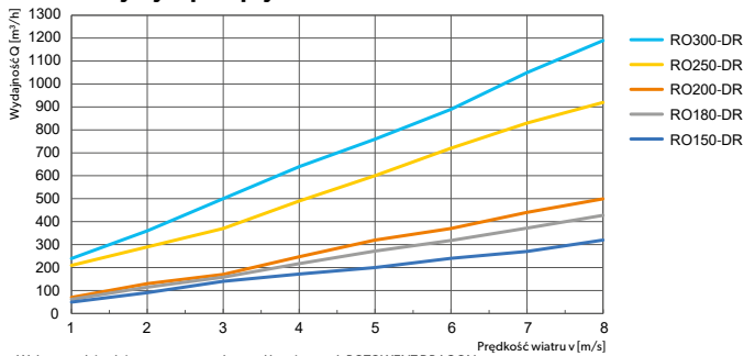
Wykres wydajności samonastawnych nasad kominowych ROTOWENT DRAGON w zależności od prędkości wiejącego wiatru bez uwzględnienia wysokości kominia. *1 [m/s] = 3.6 [km/h]
