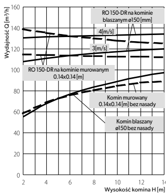
Wykres wydajności samonastawnych nasad kominowych ROTOWENT DRAGON ø150 dla kominia blaszanego i muranego, dla dwóch prędkości wiatru 3 i 4 [m/s].
