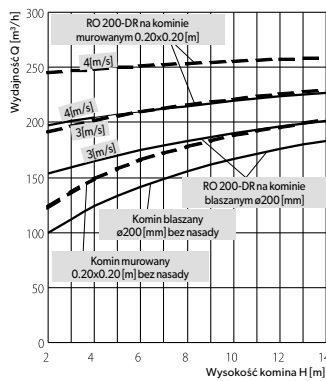
Wykres wydajności samonastawnych nasad kominowych ROTOWENT DRAGON ø200 dla kominia blaszanego i muranego, dla dwóch prędkości wiatru 3 i 4 [m/s].
